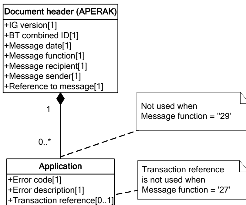
Figur 1: Fælles datamodel for APERAK
